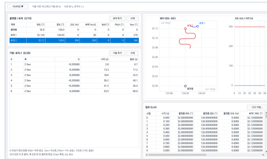
운용 화면 구성 (TargetSimUI)
