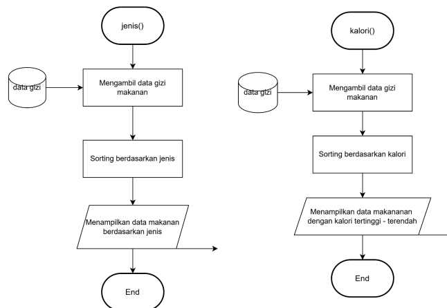
Flowchart 2.14 Menu sorting user berdasarkan jenis dan kalori
