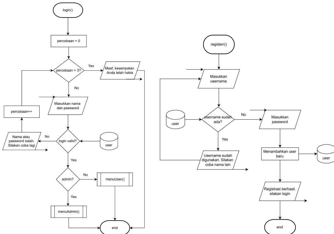
Flowchart 2.2 Menu login dan register
