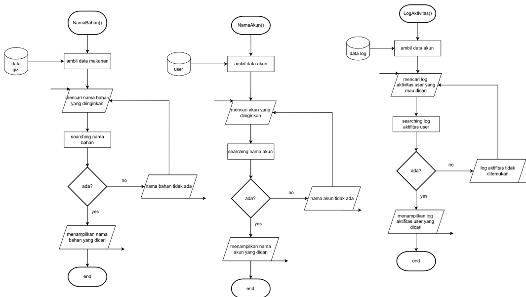
Flowchart 2.10 Menu searching nama bahan, nama akun, log aktivitas
