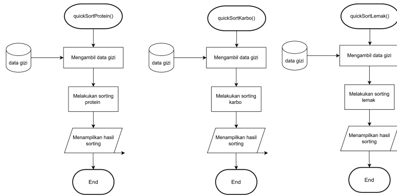
Flowchart 2.16 Menu sorting user berdasarkan makronutrisi dengan 3 pilihan
