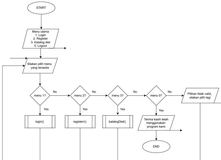
Flowchart 2.1 Menu utama
