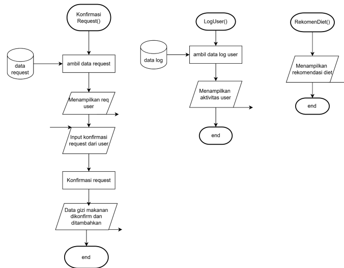
Flowchart 2.6 Menu konfirmasi request, log user dan rekomen diet
