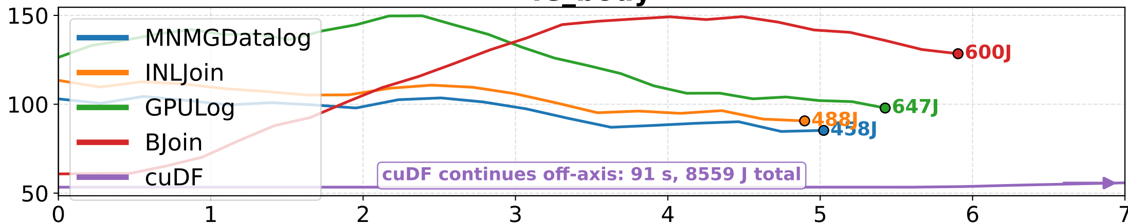
vsp
