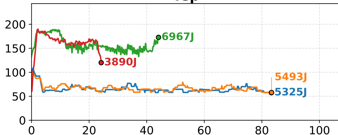
vsp
