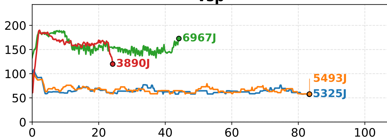
vsp
