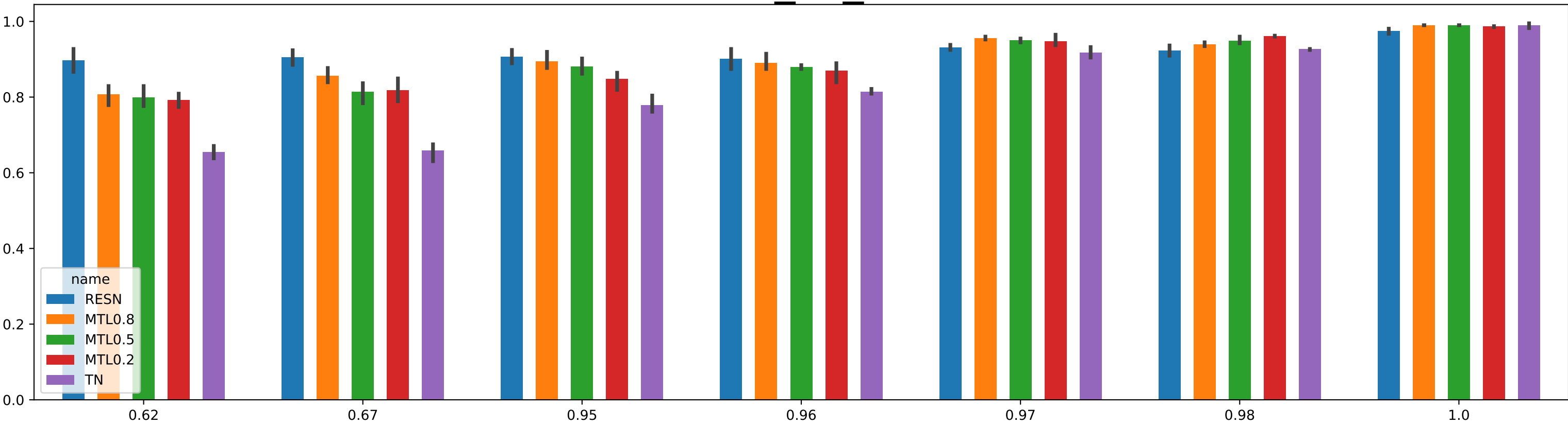
rNINO_ds_acc
