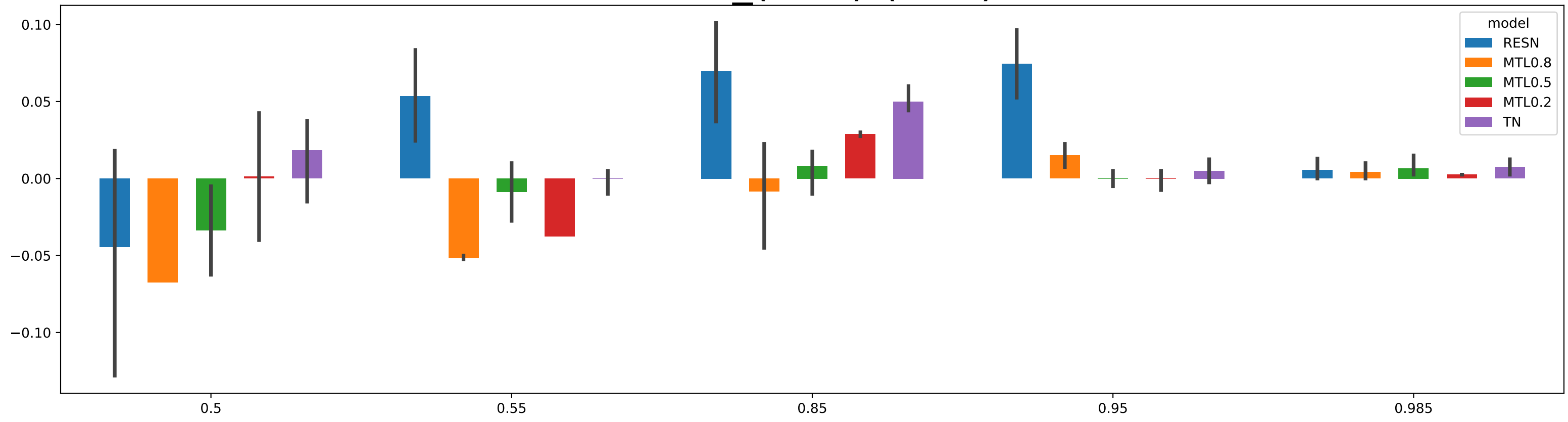
NINO_(k=5)-(k=3)
