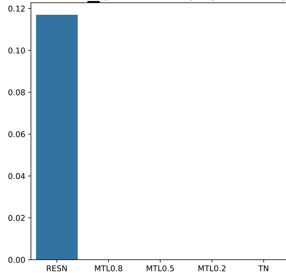
NIFO_(d=512)-(d=50)
