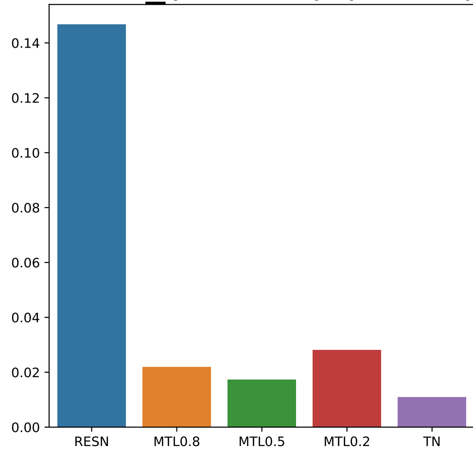
NINO_(d=512)-(d=50)
