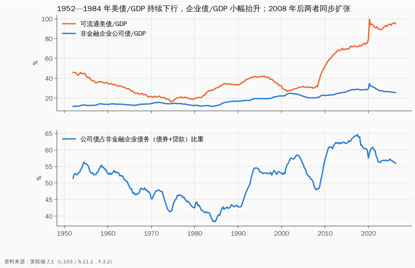
图18：1952—1984 年美债/GDP 持续下行，2008 年后美债与企业债同步扩张
