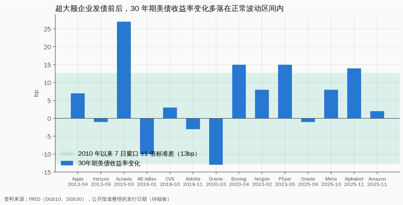
图20：超大额企业发债前后，30 年期美债收益率变化多落在正常波动区间内
