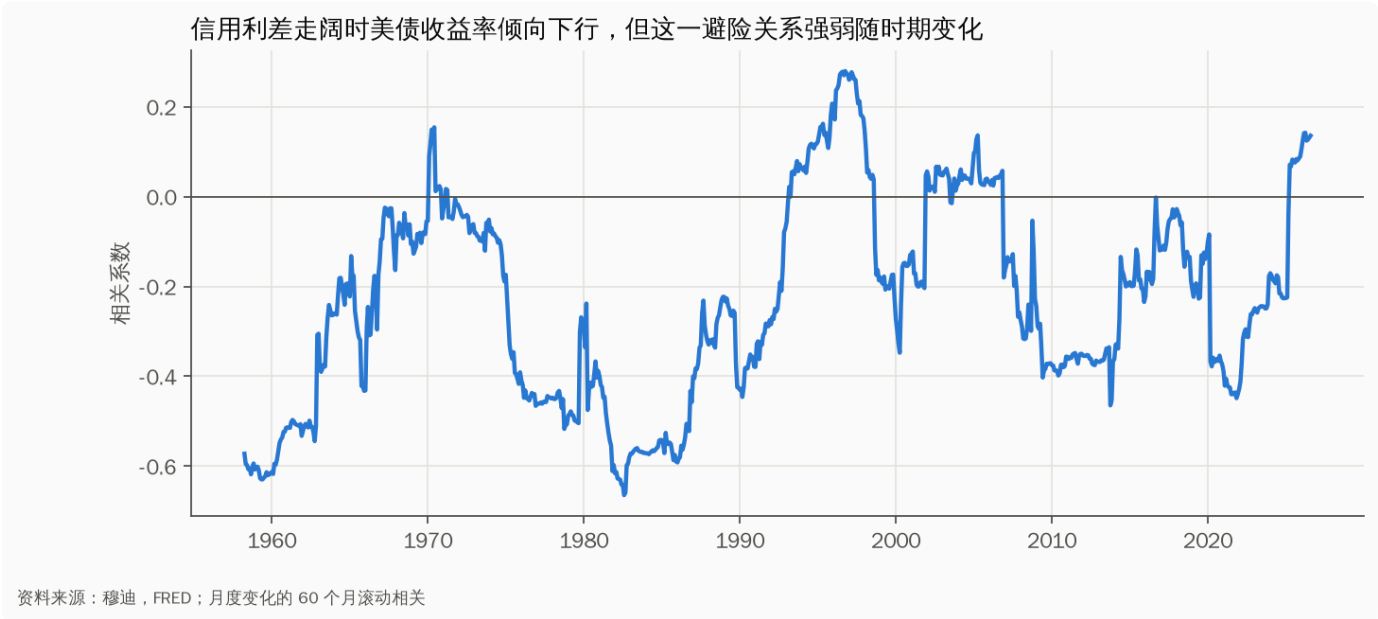
图19：信用利差走阔时美债收益率倾向下行，避险关系强弱随时期变化
