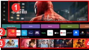
Guide
