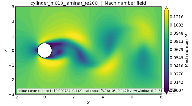
(d) Mach number.
