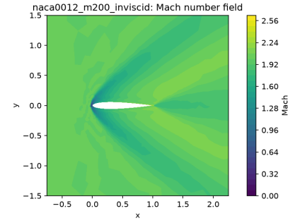
(d) Mach-number field from field_final.vtu .
