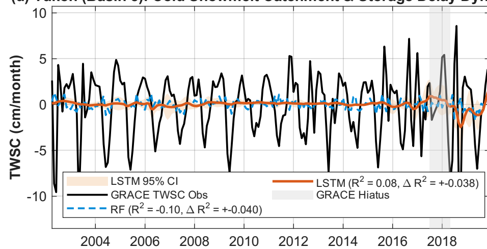
(d) Yukon (Basin 5): Cold Snowmelt Catchment & Storage Delay Dynamics
