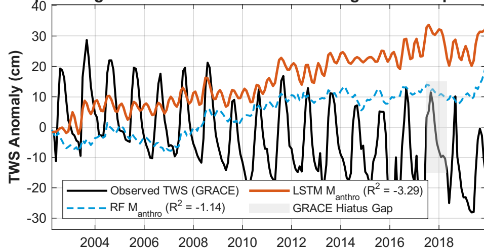
(d) Hotspot Integrated TWS Reconstruction: Ganges-Brahmaputra (Basin 51)
