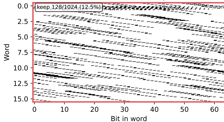
(d) Informed mask @ keep=0.125
