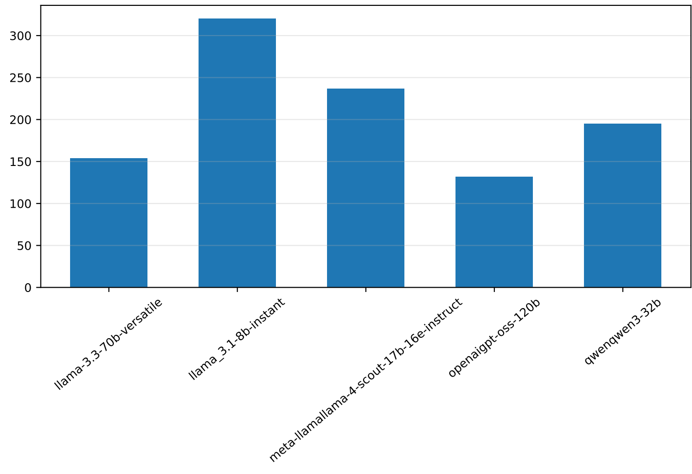
LLM calls
