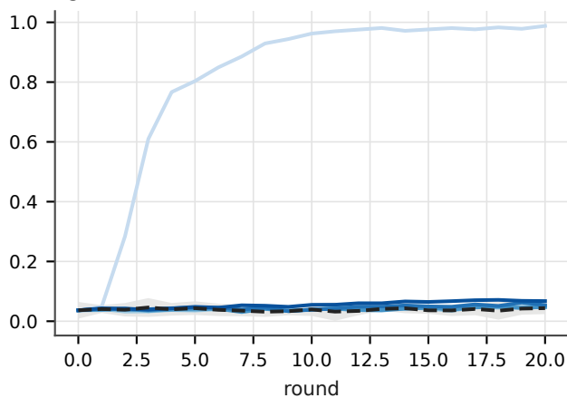
xgboost: FPR, fixed threshold
