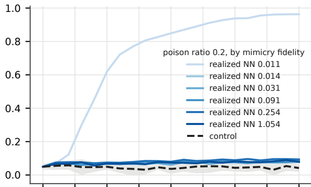
xgboost: FPR, fixed threshold
