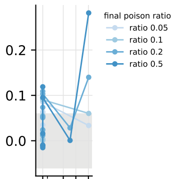
xgboost: TPR drop
