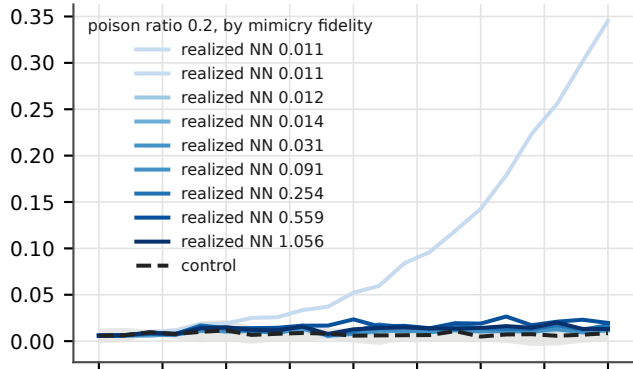
xgboost: FPR, fixed threshold
