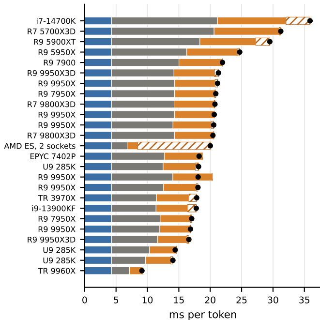
gpt-oss 11%
