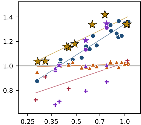
gpt-oss 11% †
