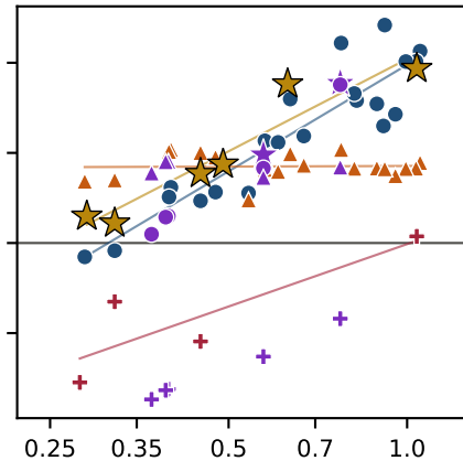
gpt-oss 25% †
