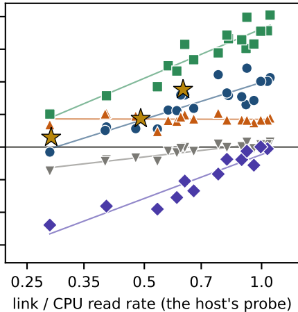
gpt-oss 25% †
