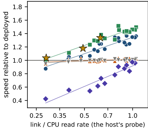
gpt-oss 11% †
