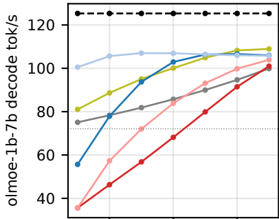
RTX 4060 8GB + DDR5-5600 (PCIe4 x8)
