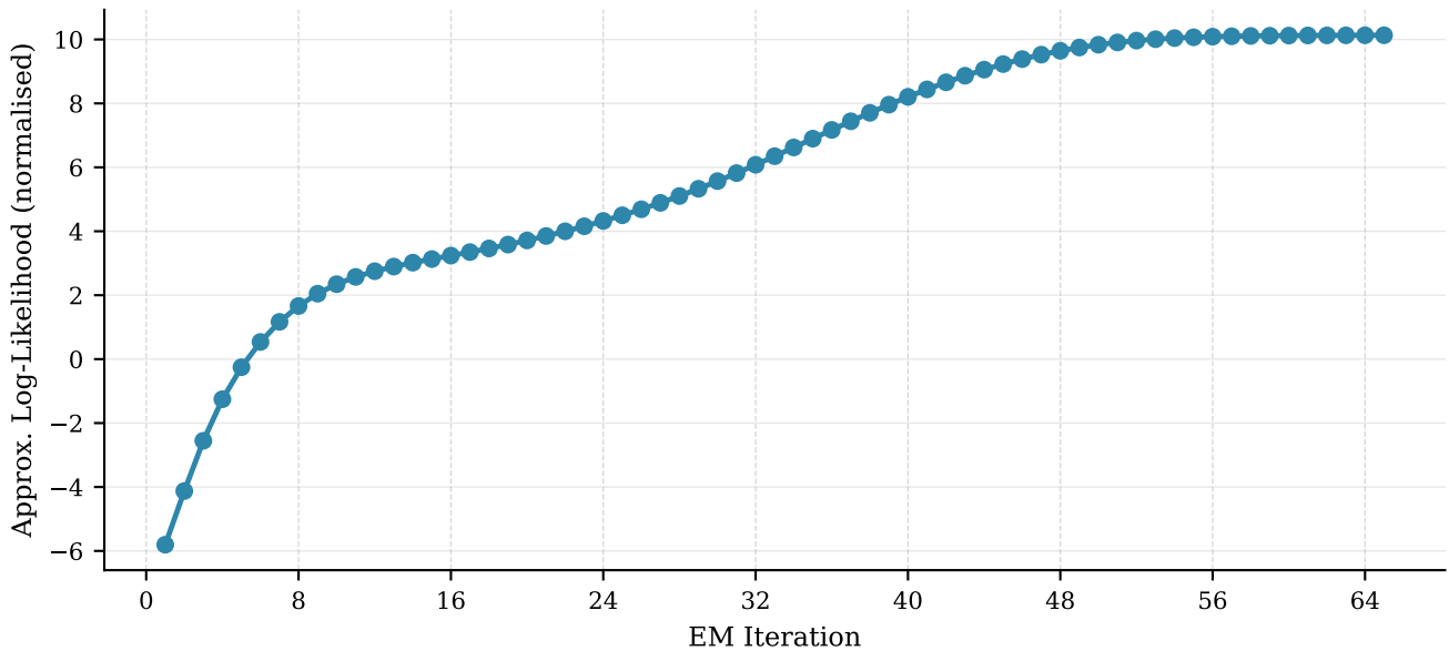
EM Convergence
