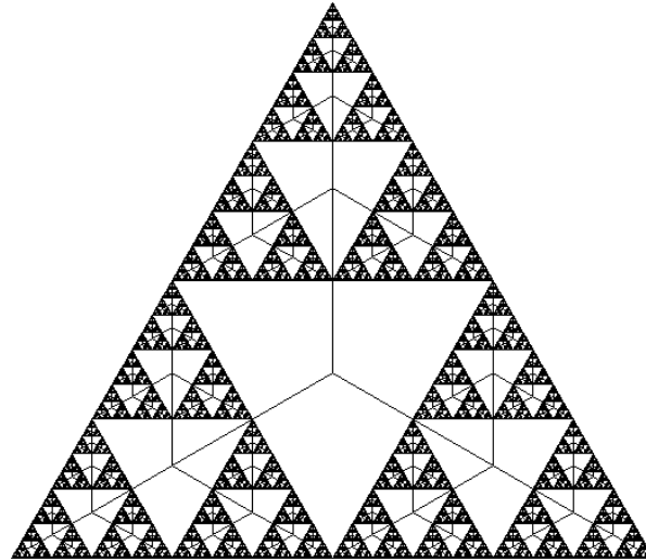
Abbildung 6.14: Sierpinski Dreieck Stufe 10
