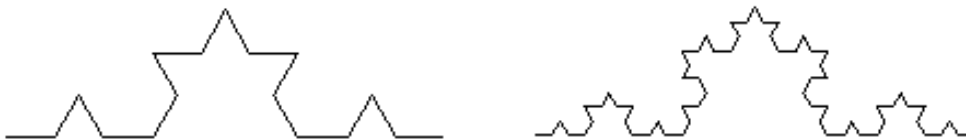
Abbildung 6.10: Kochsche Kurven der Stufe 3 und 4
