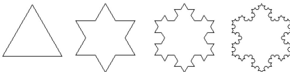
Abbildung 6.11: Kochsche Kurven werden zu Schneeflocken
