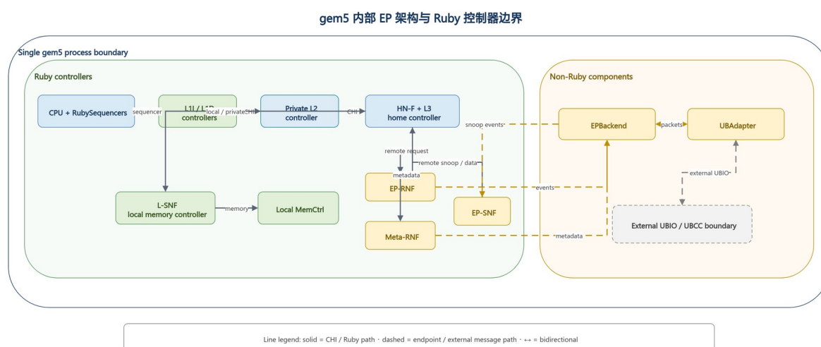
图 3-1 gem5 EP 架构。EP-RNF、EP-SNF 和 UBAdapter 位于节点内 CHI 域与 UBCC Outer 域
