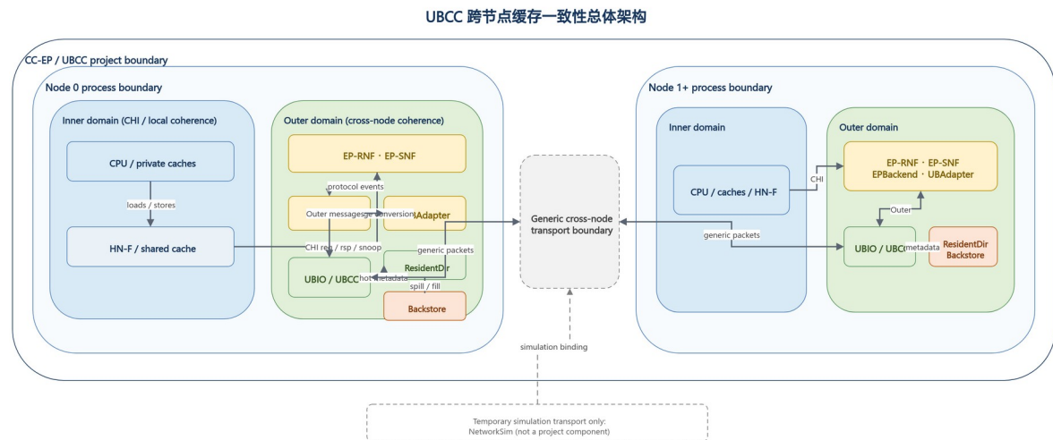
图 2-1 UBCC 总体架构。节点内请求经 EP 接入 UBCC；UBCC 根据全局目录状态完成权限
