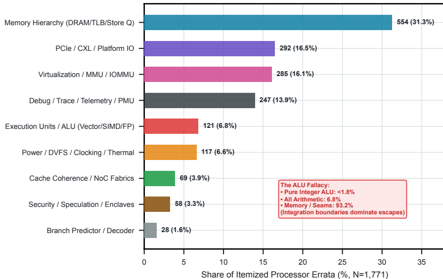
A. The 'ALU Fallacy' (Subsystem Escape Concentration)
