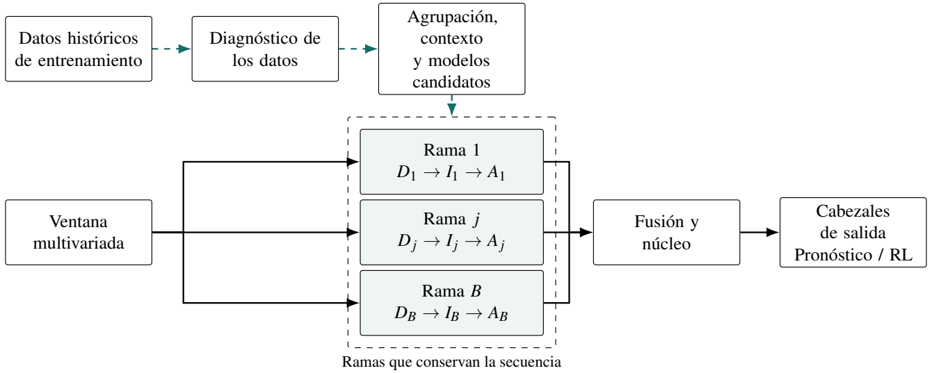
Figura 3. Arquitectura conceptual. Cada rama contiene un extractor con detector D_j e integración I_j y adaptación A_j configurables. El bloque de fusión y núcleo reúne esos dos componentes de la Figura 1.
