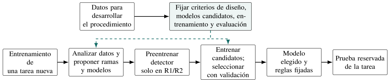
Figura 3. Separación entre desarrollo y evaluación. Durante el desarrollo se fija el procedimiento; cada tarea analiza sus datos de entrenamiento, selecciona candidatos con validación y evalúa el modelo elegido en prueba reservada.
