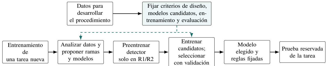
Figura 3. Separación entre desarrollo y evaluación. Durante el desarrollo se fija el procedimiento; cada tarea analiza sus datos de entrenamiento, selecciona candidatos con validación y evalúa el modelo elegido en prueba reservada.
