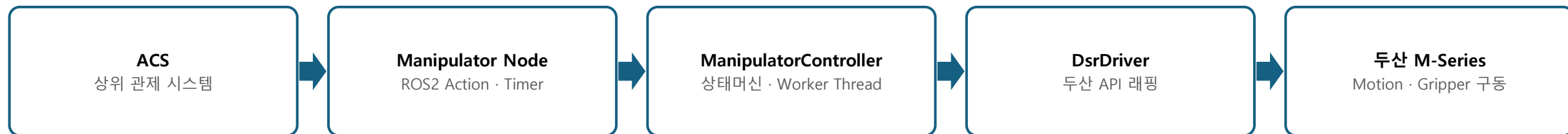
<Figure 2. 3-Layer 제어 아키텍처 — 계층별 책임 분리>
