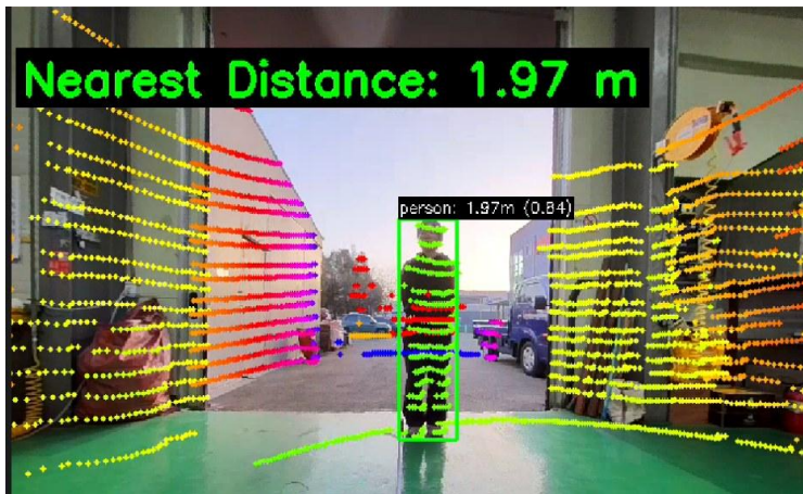
<Figure 3. LiDAR-Camera 융합 기반 실시간 객체 인식 결과>
