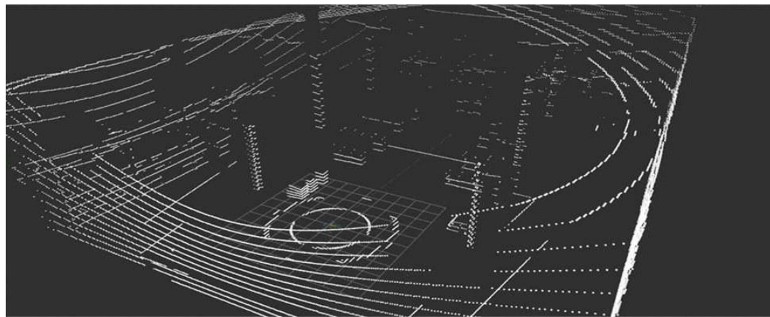
<Figure 2. base_link 기준 TF Tree 및 2대 LiDAR Point Cloud 정합 결과>
