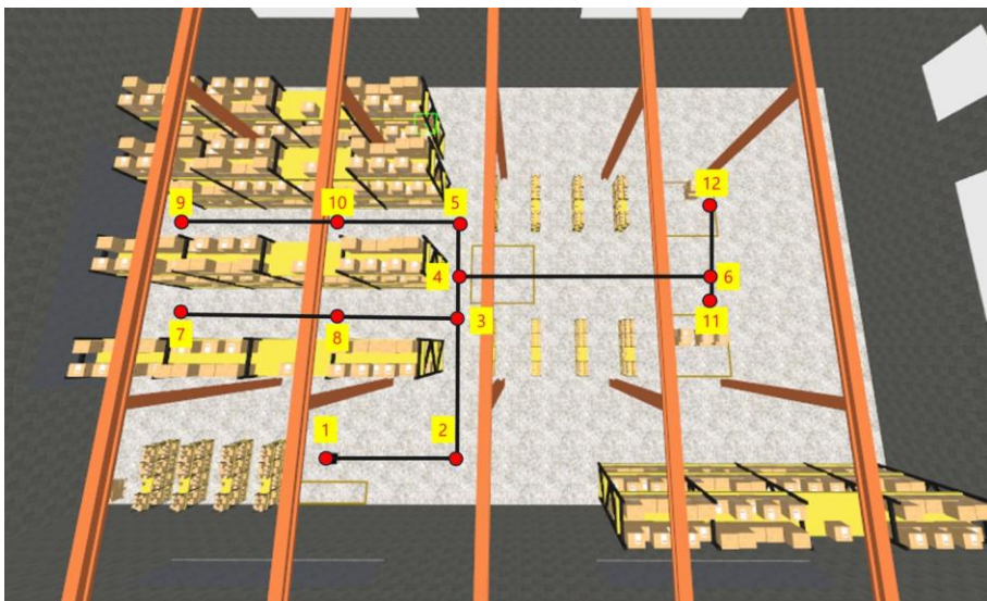
<Figure 1. HAMR3 자율주행 플랫폼 — 참고 검증 환경 및 실장비 주행>
