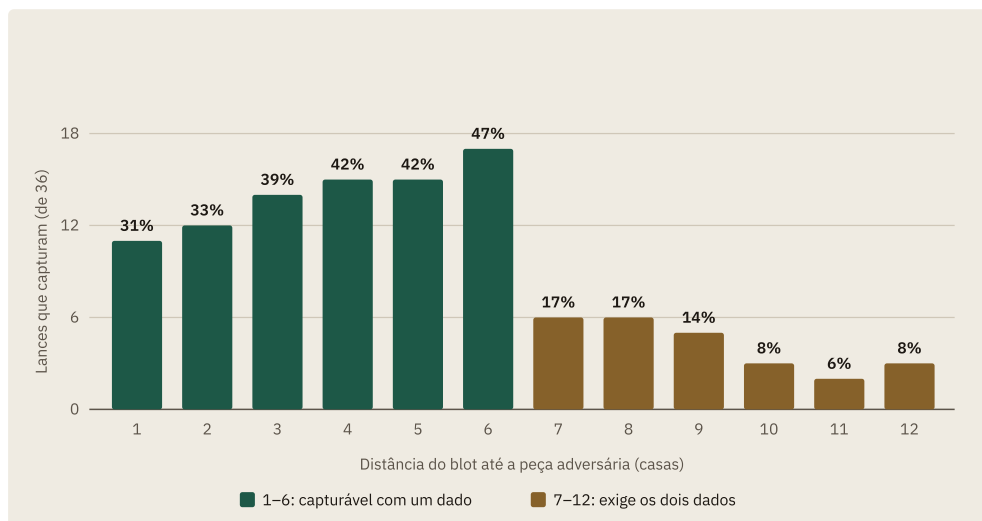
FIGURA 4.2 A probabilidade de o blot ser capturado, conforme a distância. O blot a 6 casas de distância é o que corre mais perigo; a partir de 7, o risco cai de repente. As barras mostram com quantos dos 36 lances possíveis do adversário o seu blot é capturado (se não houver pontos no caminho).
