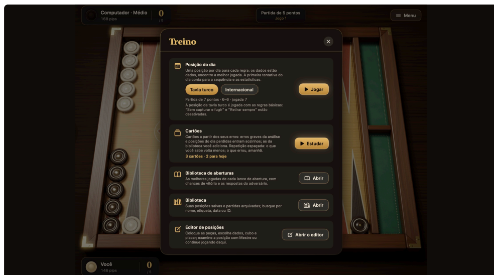
FIGURA 5.14 Cartão Treino: o bloco da posição do dia (botões de regras, duração da partida, placar e número da jogada), os cartões (resumo do baralho), a biblioteca de aberturas, a Biblioteca e o editor de posições.
