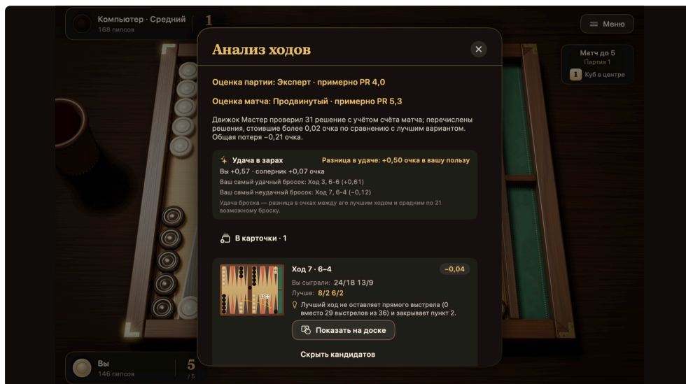
РИСУНОК 5.9 Анализ ходов.
