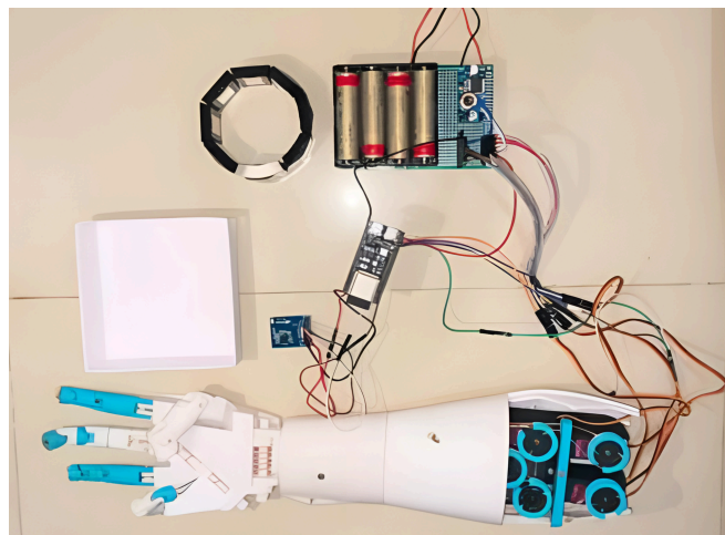
Gambar 2.3 Tangan Prostetik Mioelektrik dengan Wearable Wireless EMG Sensor yang Telah Dikembangkan Lab RES FILKOM UB Saat Ini
