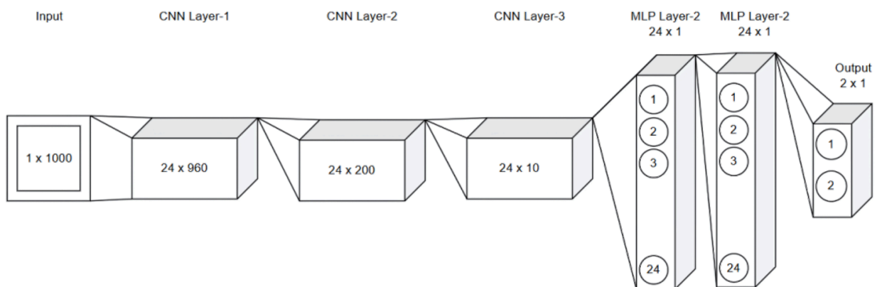
Gambar 2.4 Arsitektur 1-D CNN
