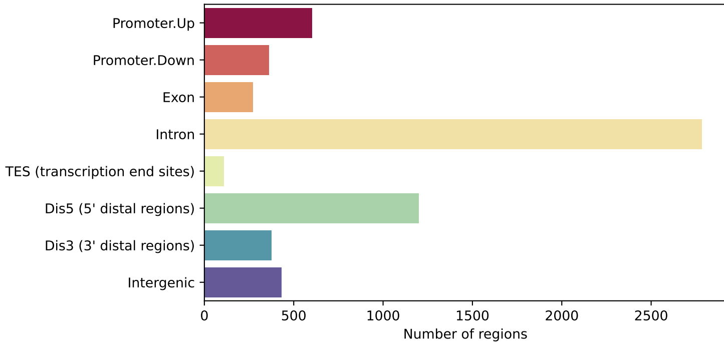
6151 regions, DownNoFDR ( p < 0.05 )
