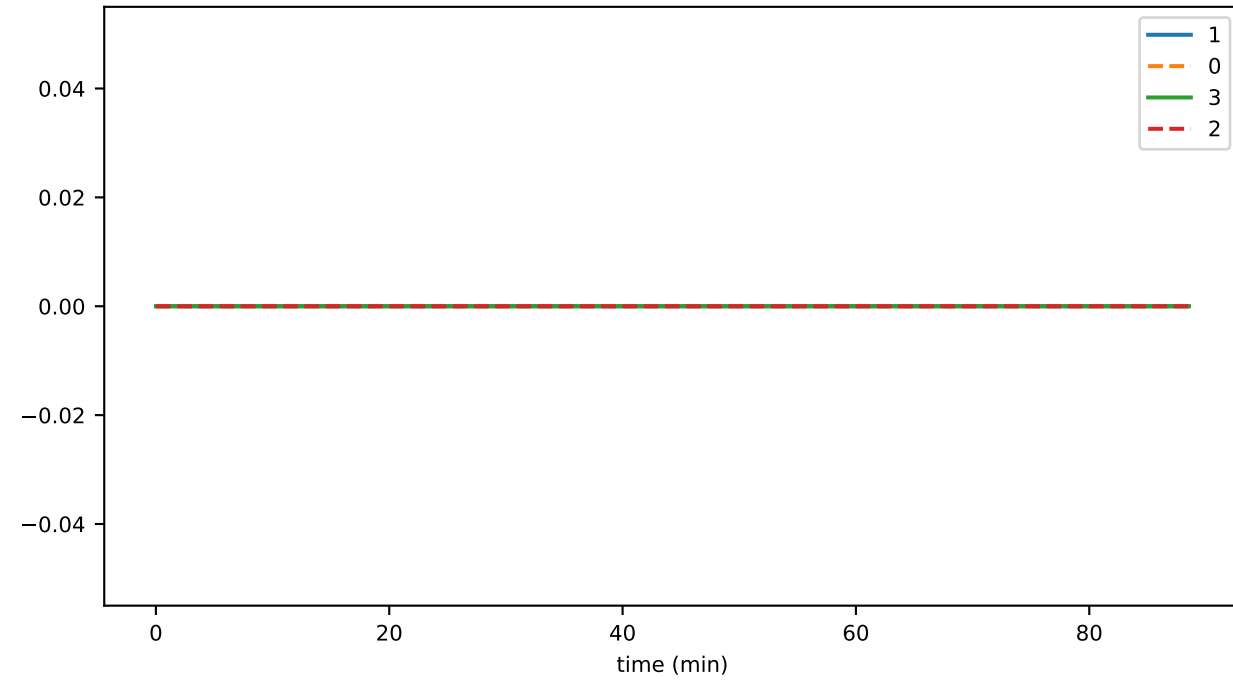
tranSubTPS
