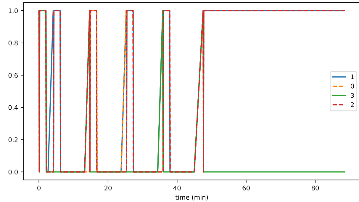
sync/secR
