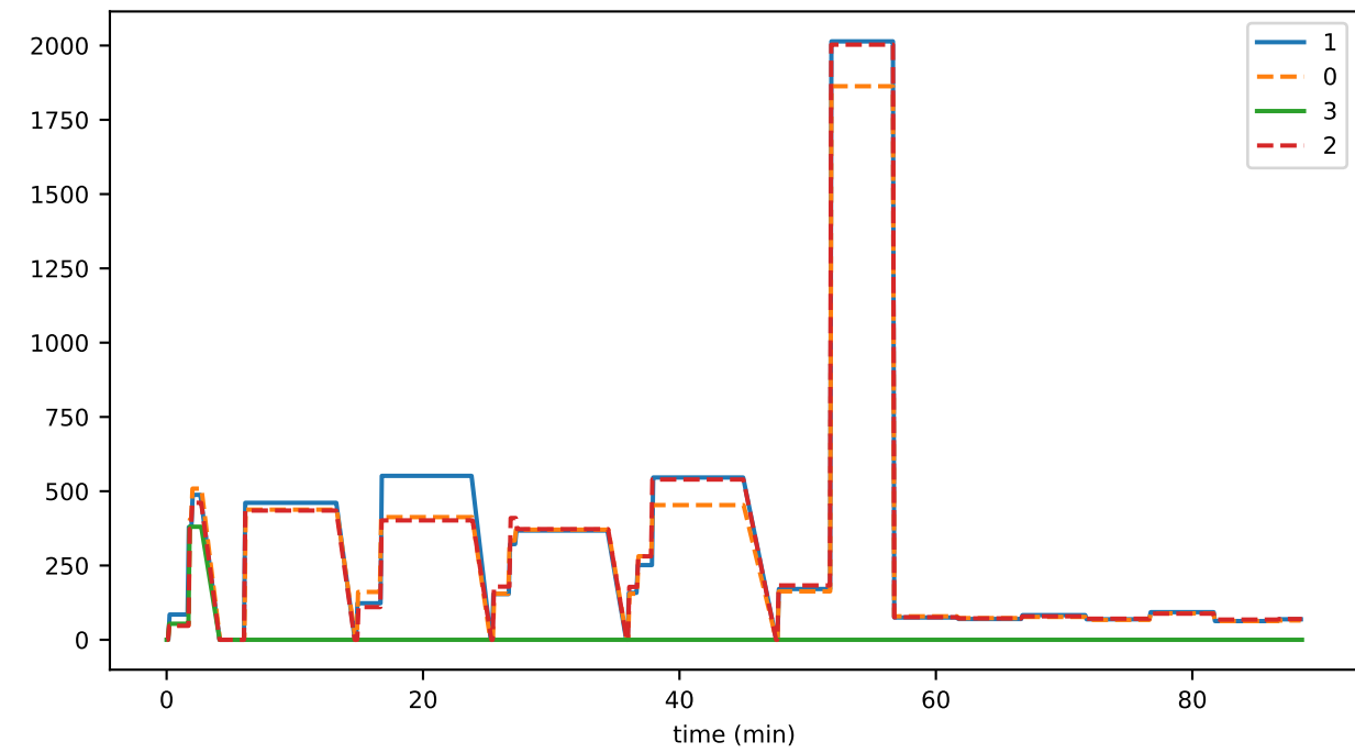
stateToDisk
