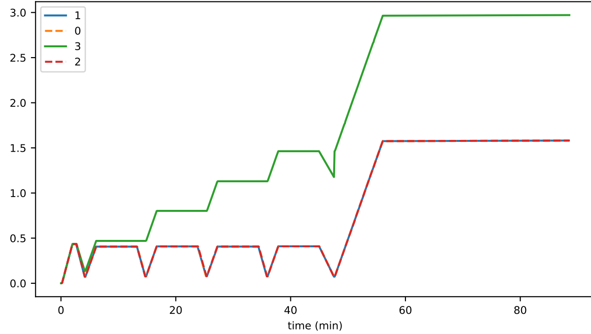
1e6 trans
