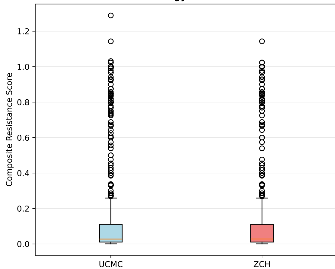
parC
