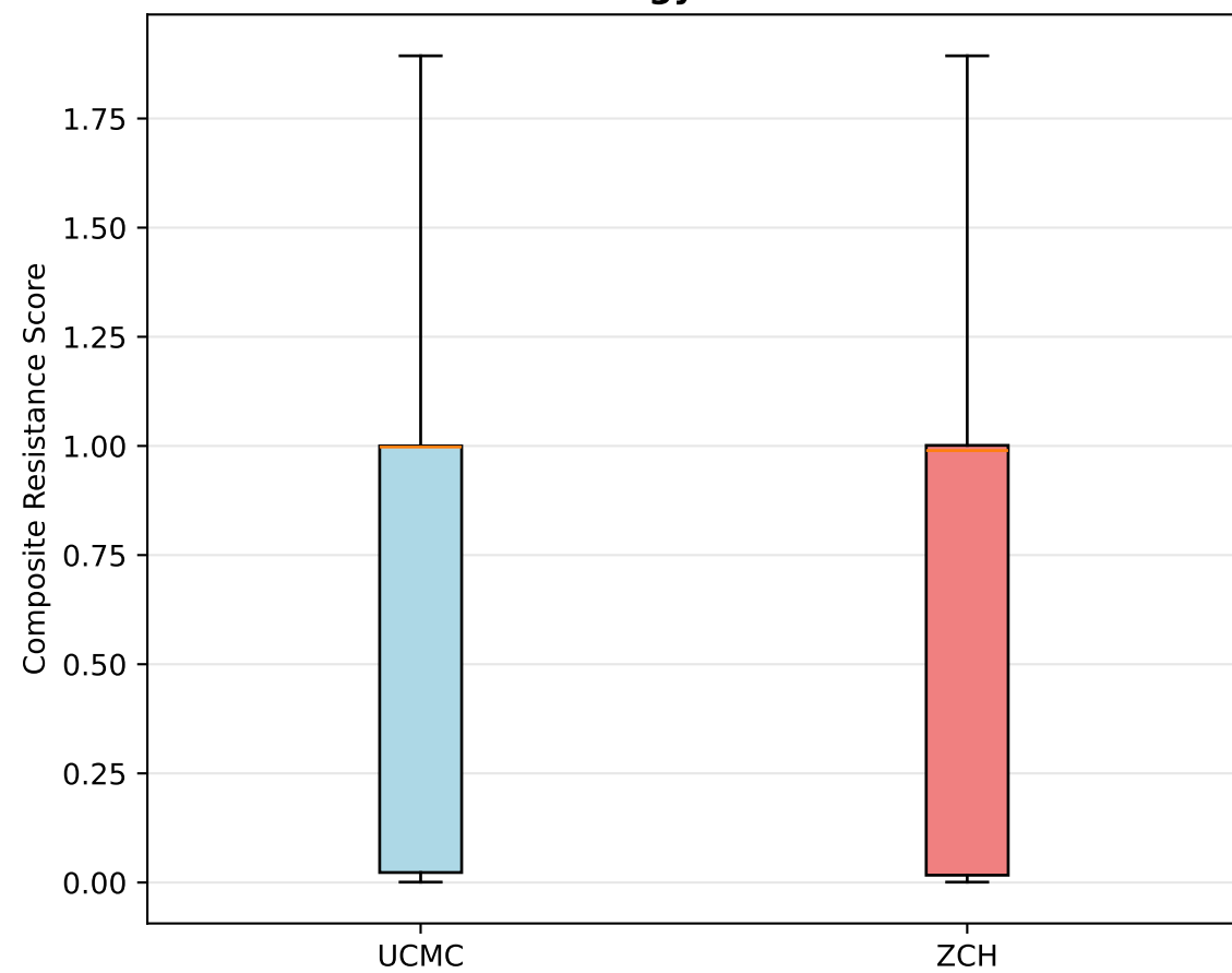
parE
