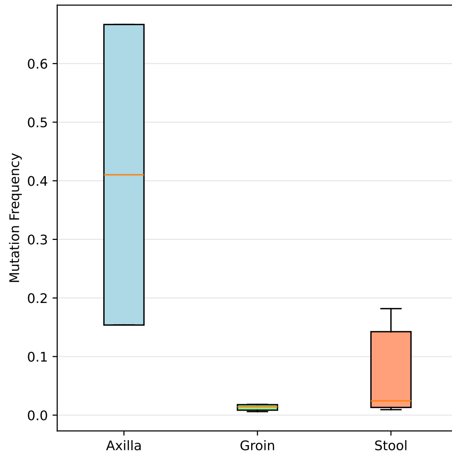
Escherichia coli gyrA 87 D->Y (FDR=4.55e-02)
