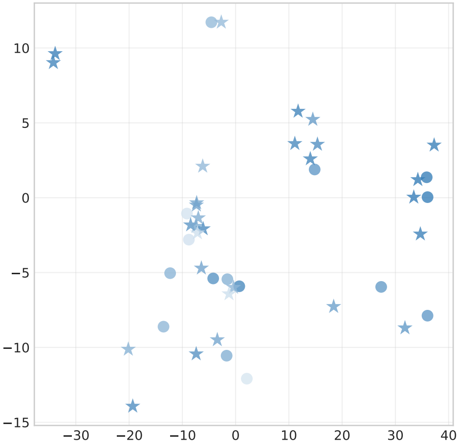
Stool (n=69)
