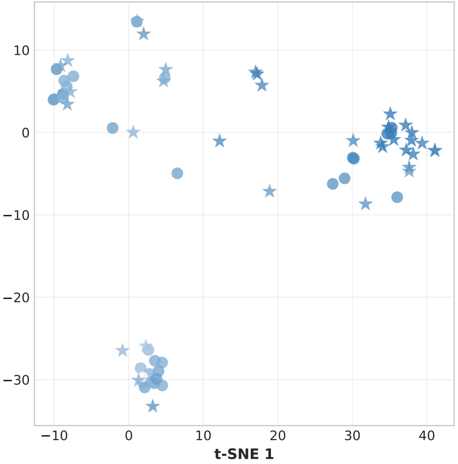
Stool (n=69)
