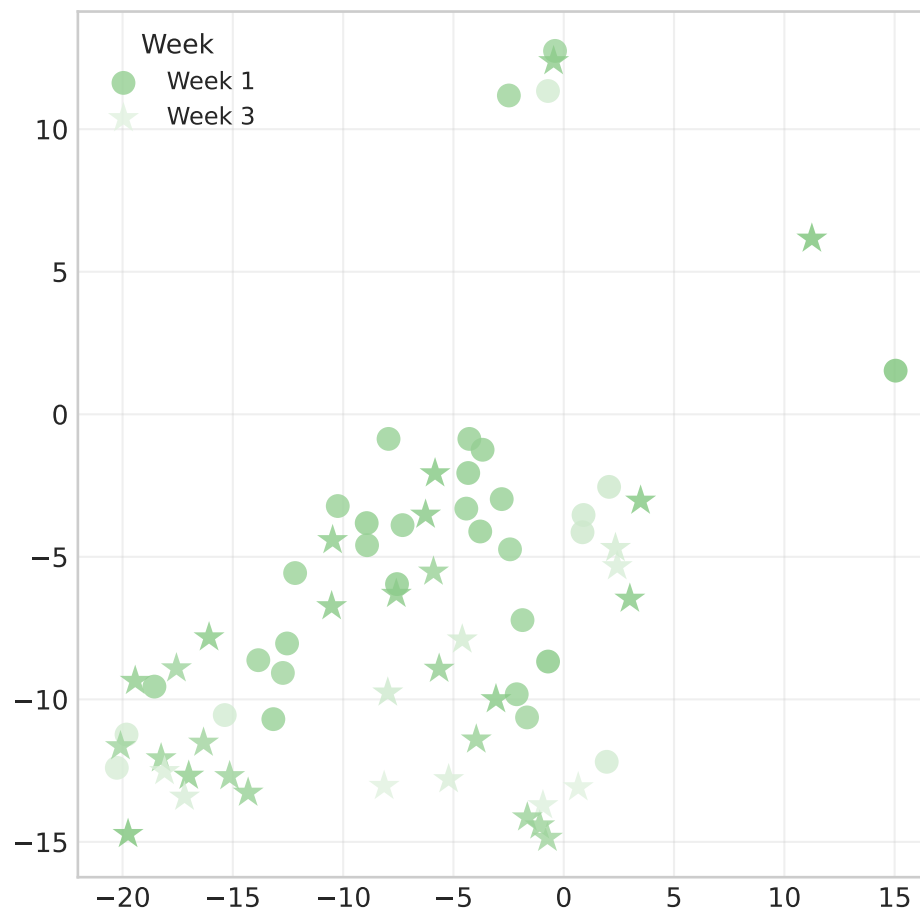
Groin (n=44)
