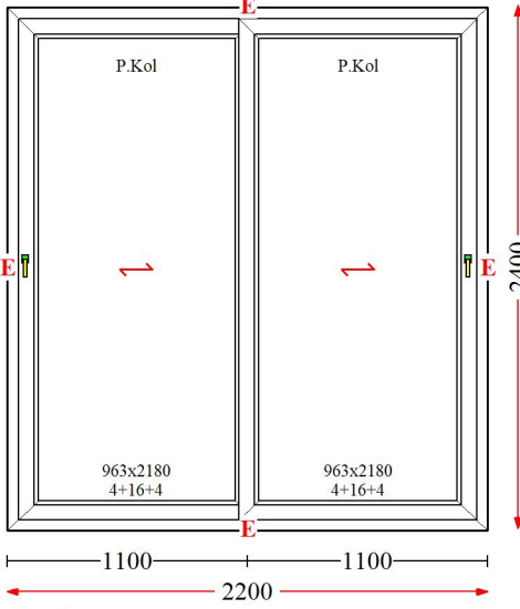
Poz : 1 / Ad : 12 - Sürme
