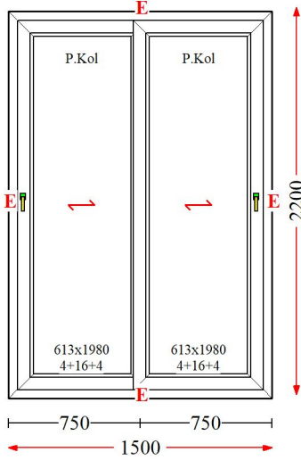
Poz : 4 / Ad : 2 - Sürme
