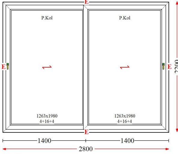
Poz : 2 / Ad : 4 - Sürme
