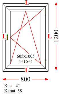
Poz : 7 / Ad : 7 - Leg.Art
