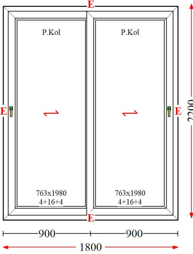
Poz : 3 / Ad : 32 - Sürme
