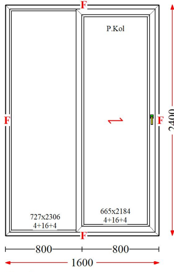
Poz : 20 / Ad : 1 - Leg.Art Poz : 21 / Ad : 2 - Leg.Poz : 22 / Ad : 4 - Sabit Sürme
