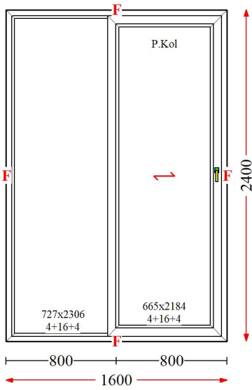
Poz : 26 / Ad : 3 - Sabit Sürme
