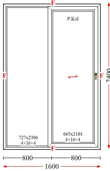
Poz : 8 / Ad : 1 - Sabit Sürme
