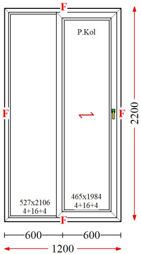
Poz : 30 / Ad : 1 - Leg.AiPoz : 31 / Ad : 2 - Leg.Poz : 32 / Ad : 1 - Sabit Sürme
