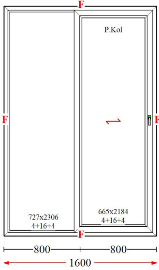
Poz : 7 / Ad : 4 - Sabit Sürme
