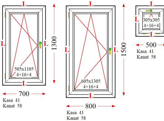
Poz : 10 / Ad : 2 - Leg.Poz : 11 / Ad : 1 - Leg.AıPoz : 12 / Ad : 1 - Poz : 13 / Ad : 1 - Sabit Sürme
