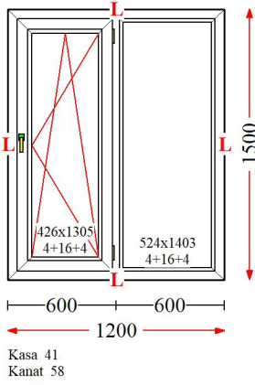
Poz : 14 / Ad : 1 - Leg.Art
