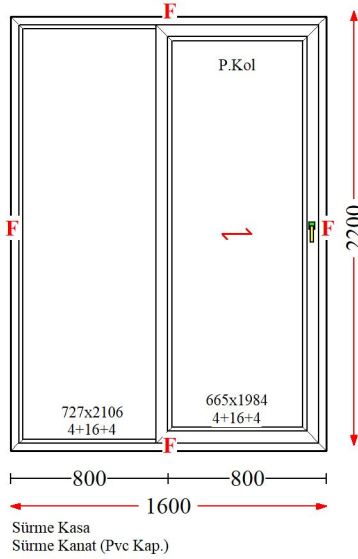
Poz : 24 / Ad : 3 - Sabit Sürme
