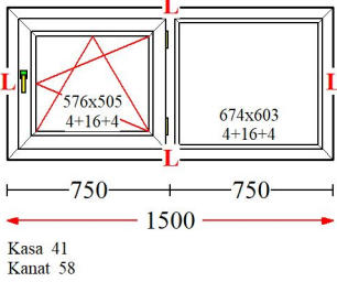
Poz : 1 / Ad : 2 - Leg.Art
