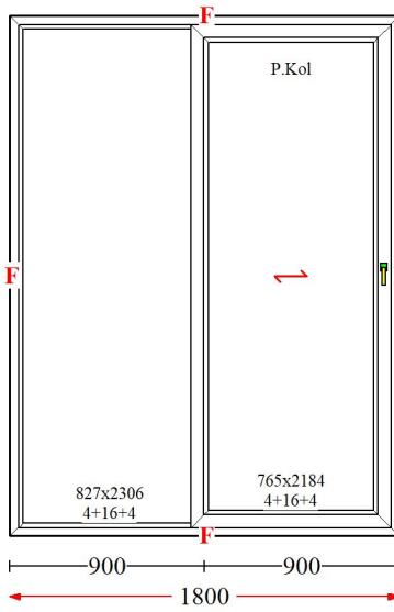
Poz : 27 / Ad : 1 - Sabit Sürme
