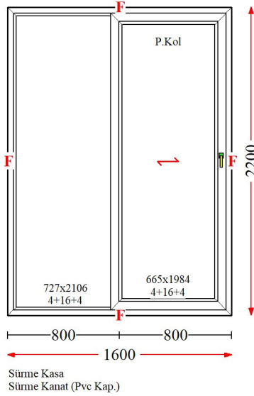
Poz : 18 / Ad : 2 - Poz : 19 / Ad : 3 - Leg.Art
