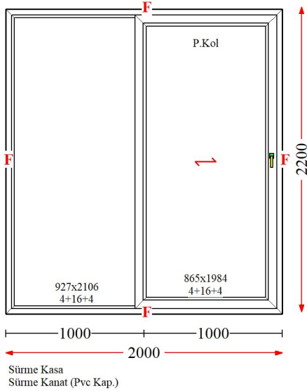
Poz : 25 / Ad : 4 - Sabit Sürme
