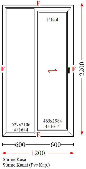
Poz : 23 / Ad : 1 - Sabit Sürme
