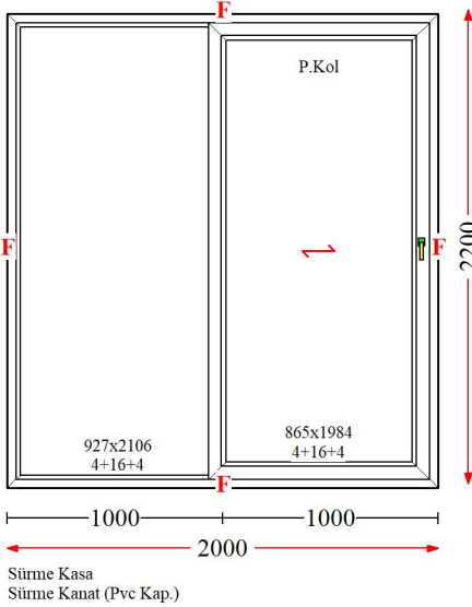
Poz : 9 / Ad : 3 - Leg.Art
