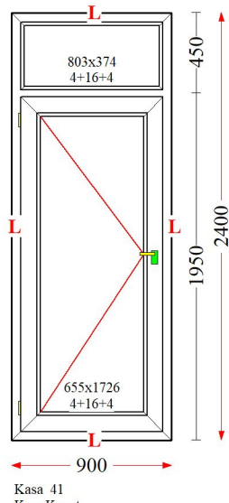
Poz : 28 / Ad : 4 - Leg.Art
