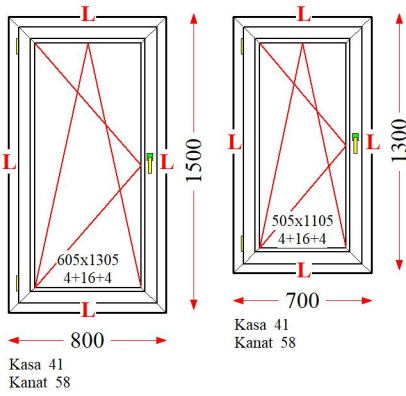
Poz : 30 / Ad : 1 - Leg.AiPoz : 31 / Ad : 2 - Leg.Poz : 32 / Ad : 1 - Sabit Sürme
