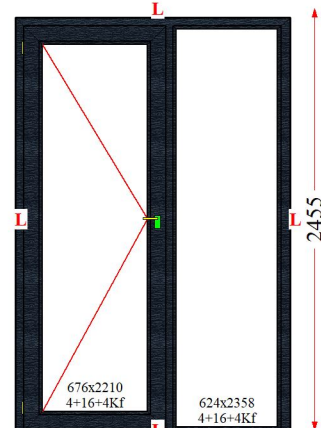
Poz : 6 / Ad : 2 - L-Poz : 7 / Ad : 2 - L-Poz : 8 / Ad : 2 - L-Poz : 9 / Ad : 2 - LegPoz : 10 / Ad : 2 - L-Poz : 11 / Ad : 2 - Leg.Art
