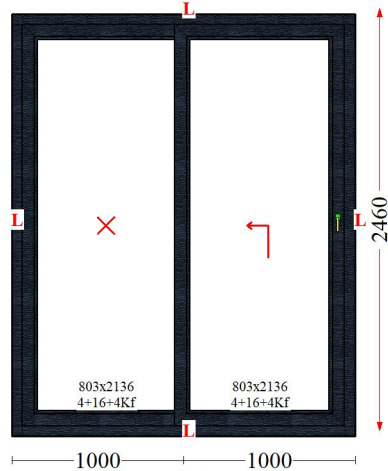
Poz : 5 / Ad : 2 - Hs 76/P
