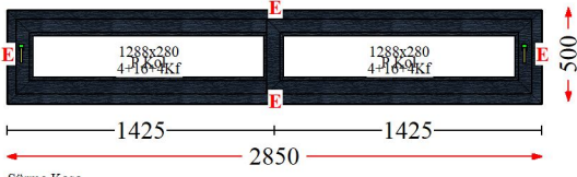
Poz : 1 / Ad : 2 - Sürme
