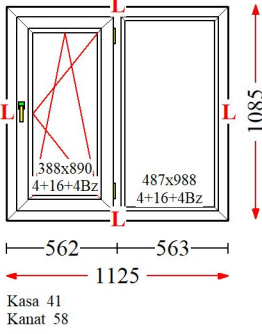
Poz : 1 / Ad : 1 - Leg.Art
