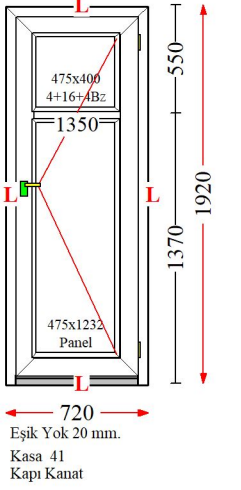
Poz : 5 / Ad : 1 - Leg.Art
