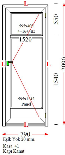
Poz : 12 / Ad : 1 - Leg.Art
