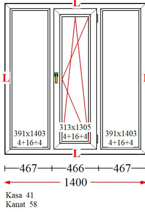
Poz : 2 / Ad : 14 - Leg.Art
