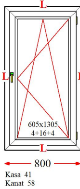
Poz : 5 / Ad : 1 - Leg.Art
