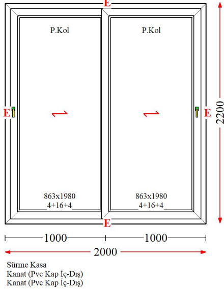
Poz : 3 / Ad : 26 - Sürme
