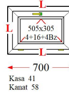
Poz : 8 / Ad : 21 - Sürme
