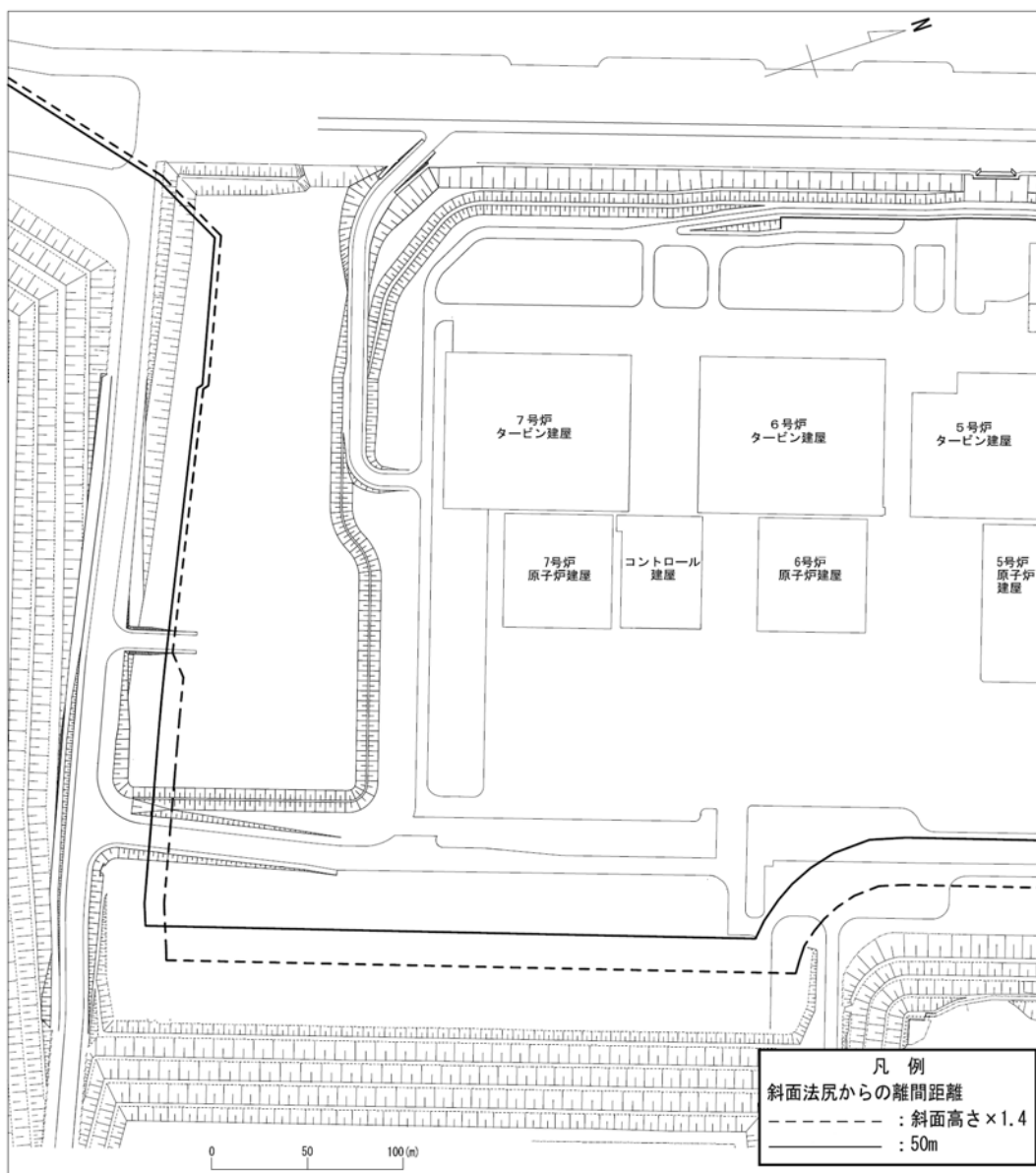
第 3. 2. 6-3 図 6 号及び 7 号炉付近平面図
