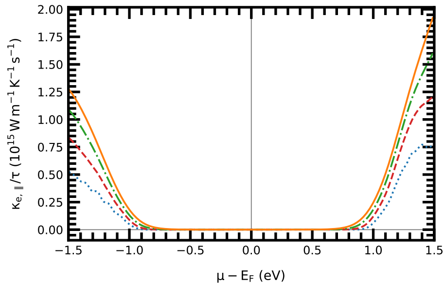
(c) Konduktivitas termal elektronik
