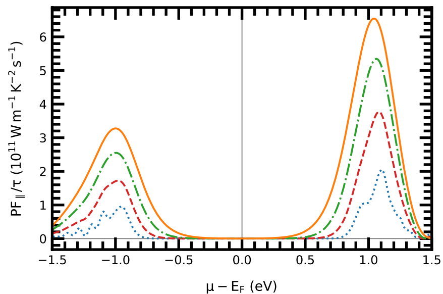
(d) Power factor
