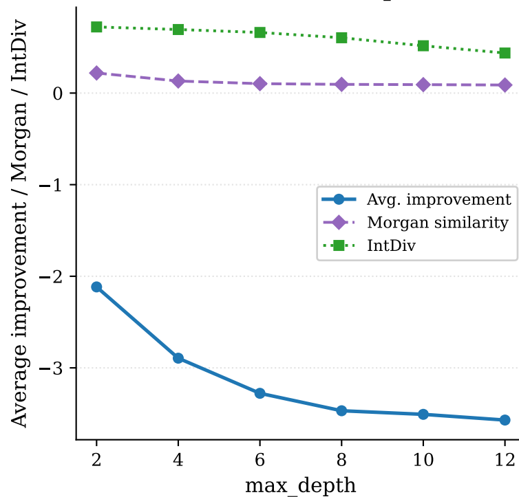
(b) LUMO(D): depth
