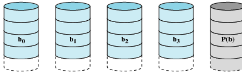
(d) RAID 3 (bit-interleaved parity)
