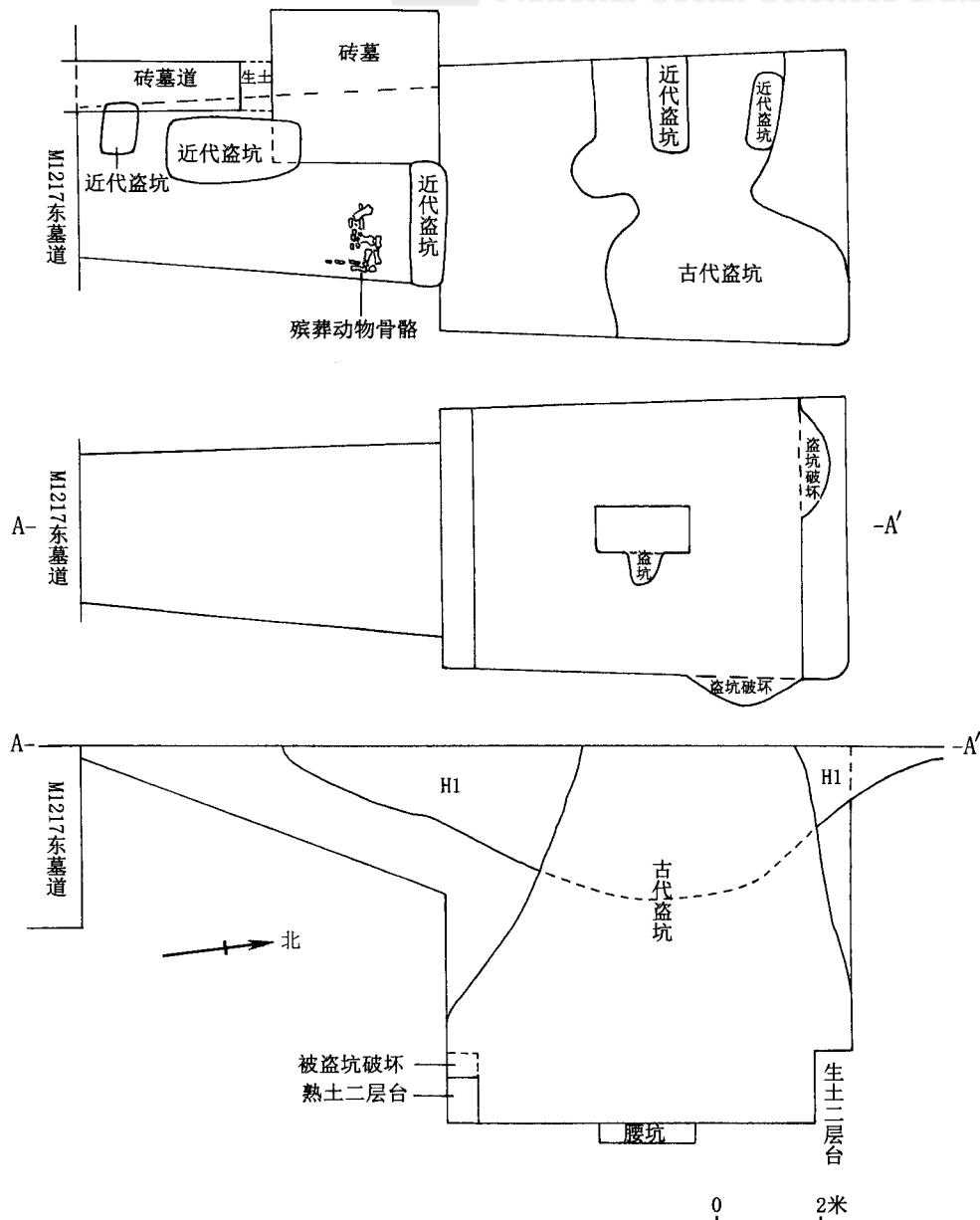
图四 78AHBM1 平、剖面图
