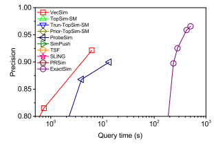
(d) webBase-2001
