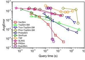
(b) Wiki-Vote
