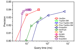
(d) HepPh
