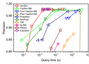
(b) Wiki-Vote
