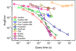
(d) HepPh
